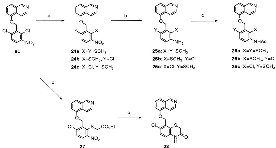
Scheme 5. Reagents: (a) \text{NaSMe} , DMF; (b) \text{NH}_2\text{NH}_2 , \text{FeCl}_3 ; (c) \text{Ac}_2\text{O} , \text{ClCH}_2\text{CH}_2\text{Cl} ; (d) \text{HSCH}_2\text{CO}_2\text{Et} , \text{Et}_3\text{N} , DMF; (e) \text{Fe} , \text{NH}_4\text{Cl} , \text{EtOH}-\text{H}_2\text{O} .
