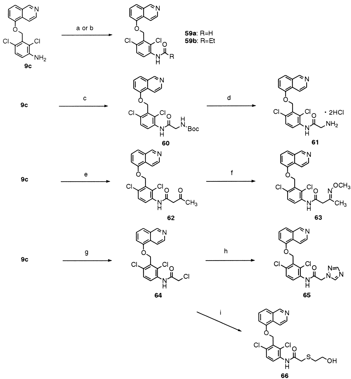
Scheme 10. Reagents: (a) \text{HCO}_2\text{H} , \text{Ac}_2\text{O} ; (b) (\text{EtCO})_2\text{O} , DMAP, Py; (c) Boc-Gly, HOBT, WSCD-HCl, \text{CH}_2\text{Cl}_2 ; (d) HCl, AcOEt; (e) diketene, \text{ClCH}_2\text{CH}_2\text{Cl} ; (f) \text{NH}_2\text{OCH}_3\cdot\text{HCl} , EtOH; (g) (\text{ClCH}_2\text{CO})_2\text{O} , \text{ClCH}_2\text{CH}_2\text{Cl} ; (h) 1,2,4-triazole Na-salt, DMF; (i) \text{HSCH}_2\text{CH}_2\text{OH} , \text{Et}_3\text{N} , \text{CH}_2\text{Cl} , DMF.
