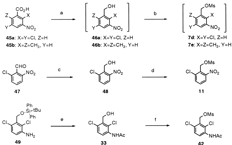
Scheme 8. Reagents: (a) \text{NaBH}_4 , \text{BF}_3\cdot\text{Et}_2\text{O} , THF; (b) \text{MsCl} , \text{Et}_3\text{N} , \text{AcOEt} ; (c) \text{NaBH}_4 , EtOH; (d) \text{MsCl} , \text{Et}_3\text{N} , \text{AcOEt-CH}_2\text{Cl}_2 ; (e) (1) \text{Ac}_2\text{O} , Py, DMAP, \text{CH}_2\text{Cl}_2 , (2) TBAF, THF; (f) \text{MsCl} , \text{Et}_3\text{N} , \text{AcOEt-CH}_2\text{Cl}_2 .
