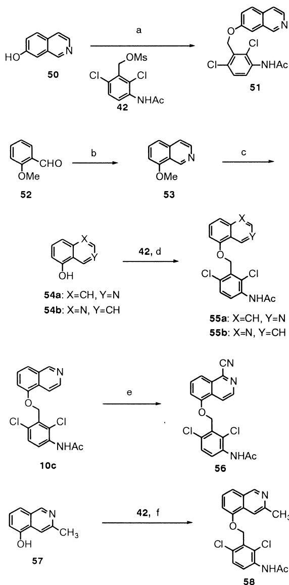
Scheme 9. Reagents: (a) NaH, DMF; (b) (1) (\text{MeO})_2\text{CHCH}_2\text{NH}_2 , benzene, (2) \text{ClCO}_2\text{Et} , \text{P}(\text{OMe})_3 , THF, (3) \text{TiCl}_4 , \text{CH}_2\text{Cl}_2 ; (c) \text{BBR}_3 , \text{CH}_2\text{Cl}_2 ; (d) NaH, DMF; (e) (1) p -TsCl, KCN, \text{CH}_2\text{Cl}_2 - \text{H}_2\text{O} , (2) DBU, THF; (f) NaH, DMF.
