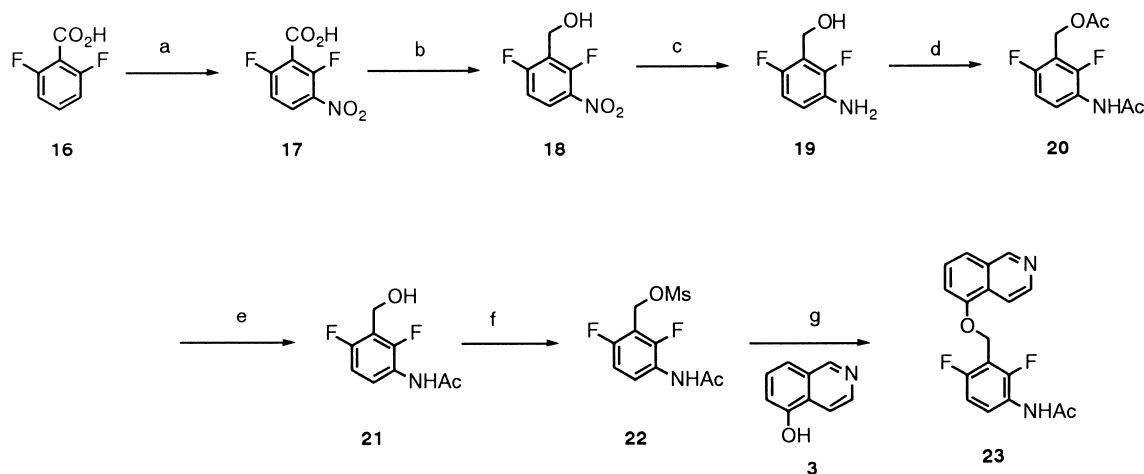
Scheme 4. Reagents: (a) \text{HNO}_3 ; (b) \text{NaBH}_4 , \text{BF}_3 \cdot \text{Et}_2\text{O} , THF; (c) \text{H}_2 , Pd/C, \text{AcOEt} ; (d) (1) \text{Ac}_2\text{O} , \text{Et}_3\text{N} , \text{ClCH}_2\text{CH}_2\text{Cl} , (2) pyrrolidine, \text{EtOH} ; (e) 1 \text{N-NaOH} , \text{MeOH} ; (f) \text{MsCl} , \text{Et}_3\text{N} , \text{CH}_2\text{Cl}_2 ; (g) \text{NaH} , DMF.
