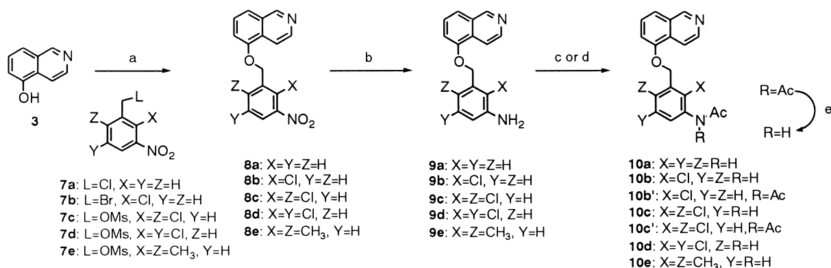
Scheme 2. Reagents: (a) NaH, DMF; (b) NH 2 NH 2 , FeCl 3 , H 2 O–MeOH; (c) Ac 2 O, Py, DMAP; (d) Ac 2 O, ClCH 2 CH 2 Cl; (e) pyrrolidine, EtOH.
