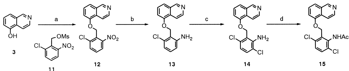
Scheme 3. Reagents: (a) NaH, DMF; (b) NH 2 NH 2 , FeCl 3 , H 2 O–MeOH; (c) NCS, CHCl 3 ; (d) Ac 2 O, ClCH 2 CH 2 Cl.
